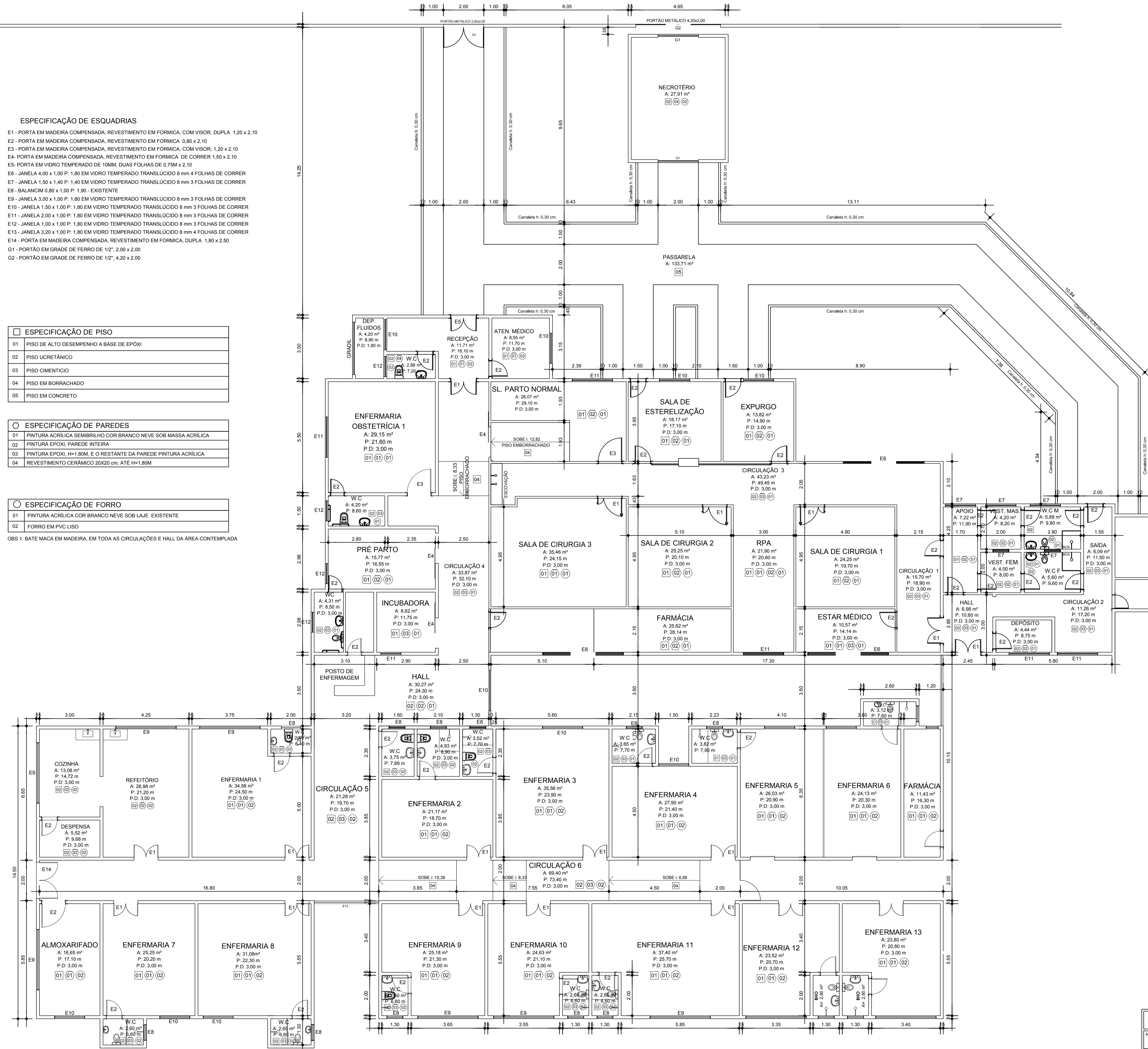
PLANTA BAIXA PAVIMENTO TÉRREO ESC 1/100
