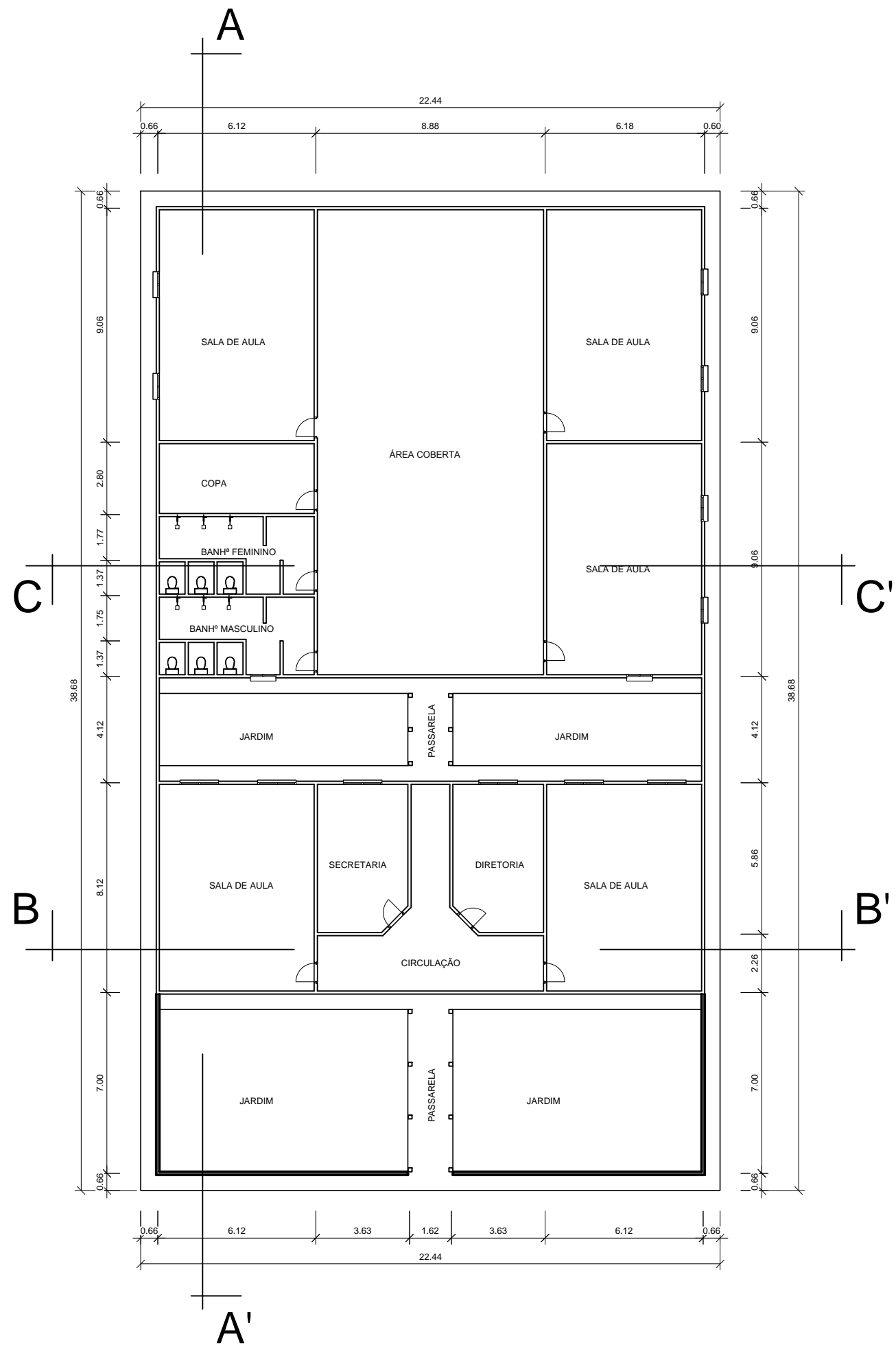
Planta baixa
