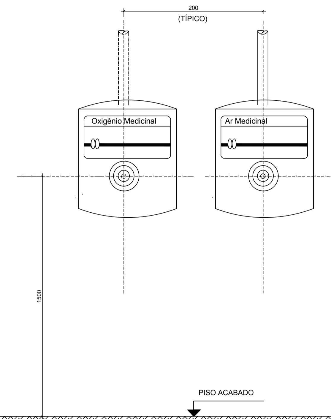
DETALHE SEQUÊNCIA DE MONTAGEM DO POSTO DE CONSUMO S/ ESCALA
