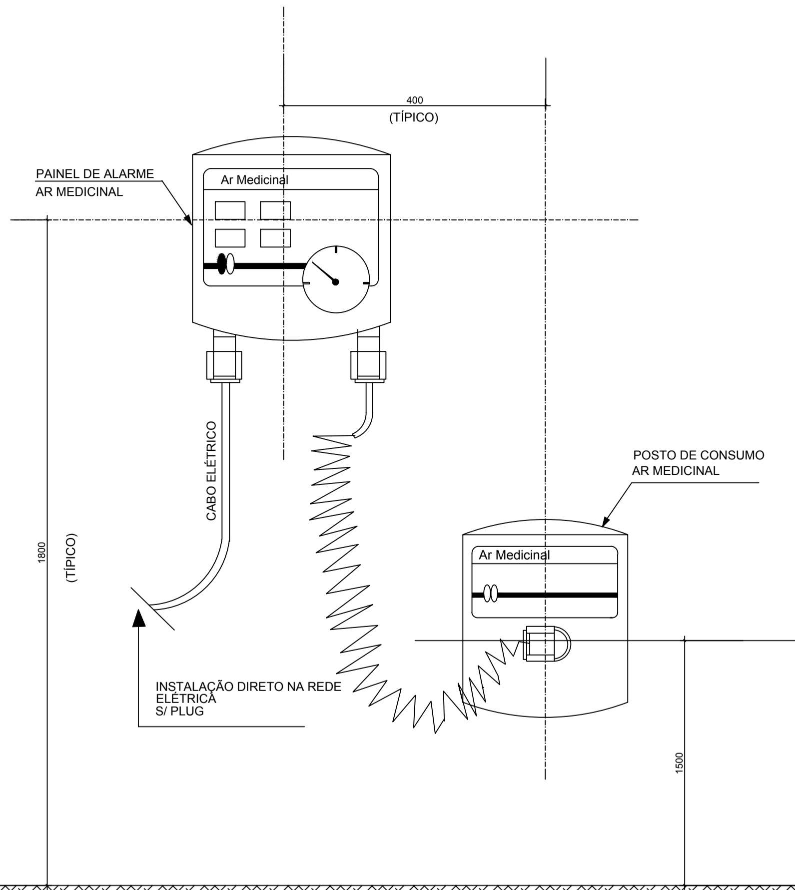
DETALHE SEQUÊNCIA DE MONTAGEM DO PAINEL DE ALARME S/ ESCALA
