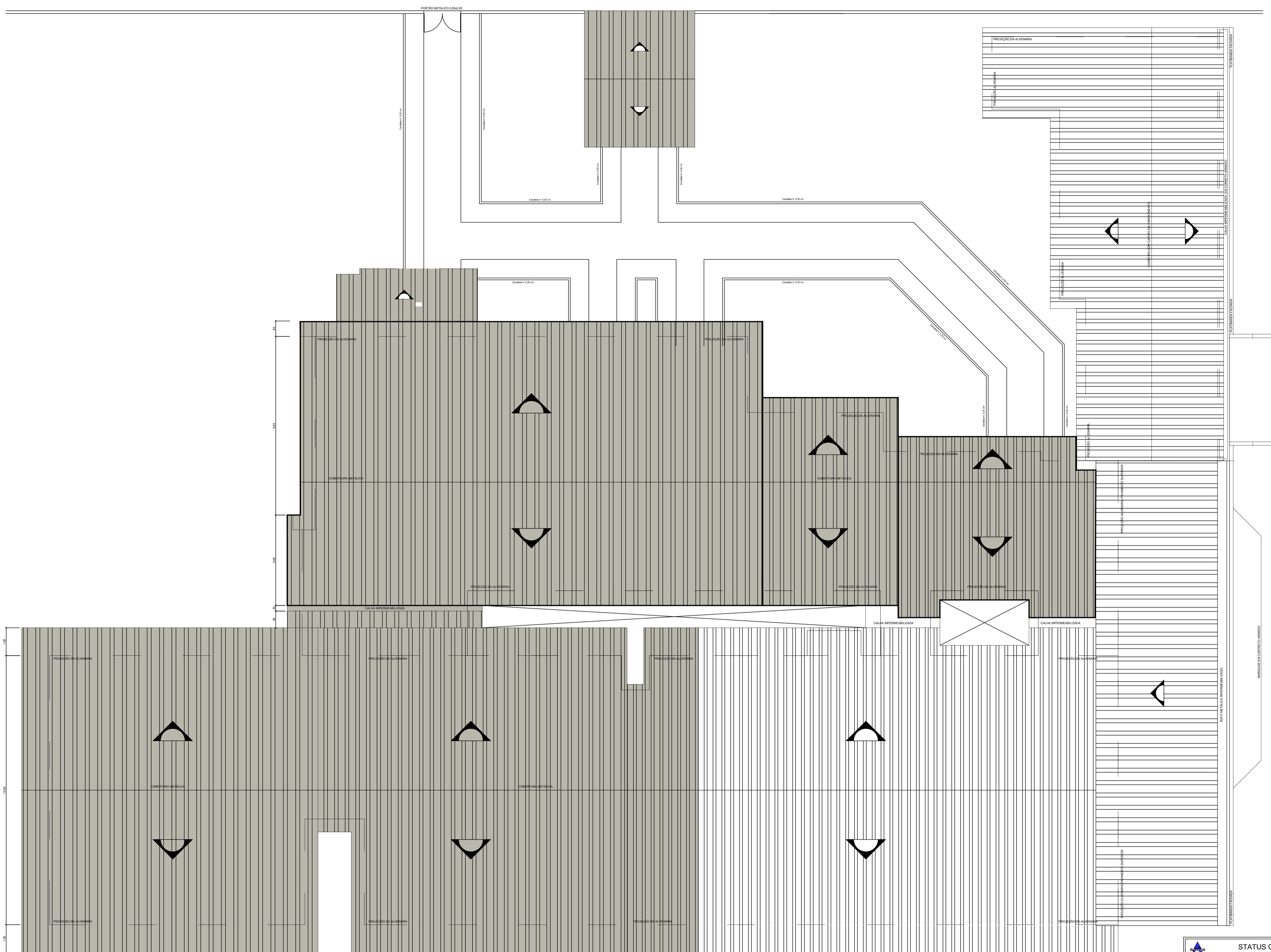
PLANTA DE COBERTURA ESC 1/100
