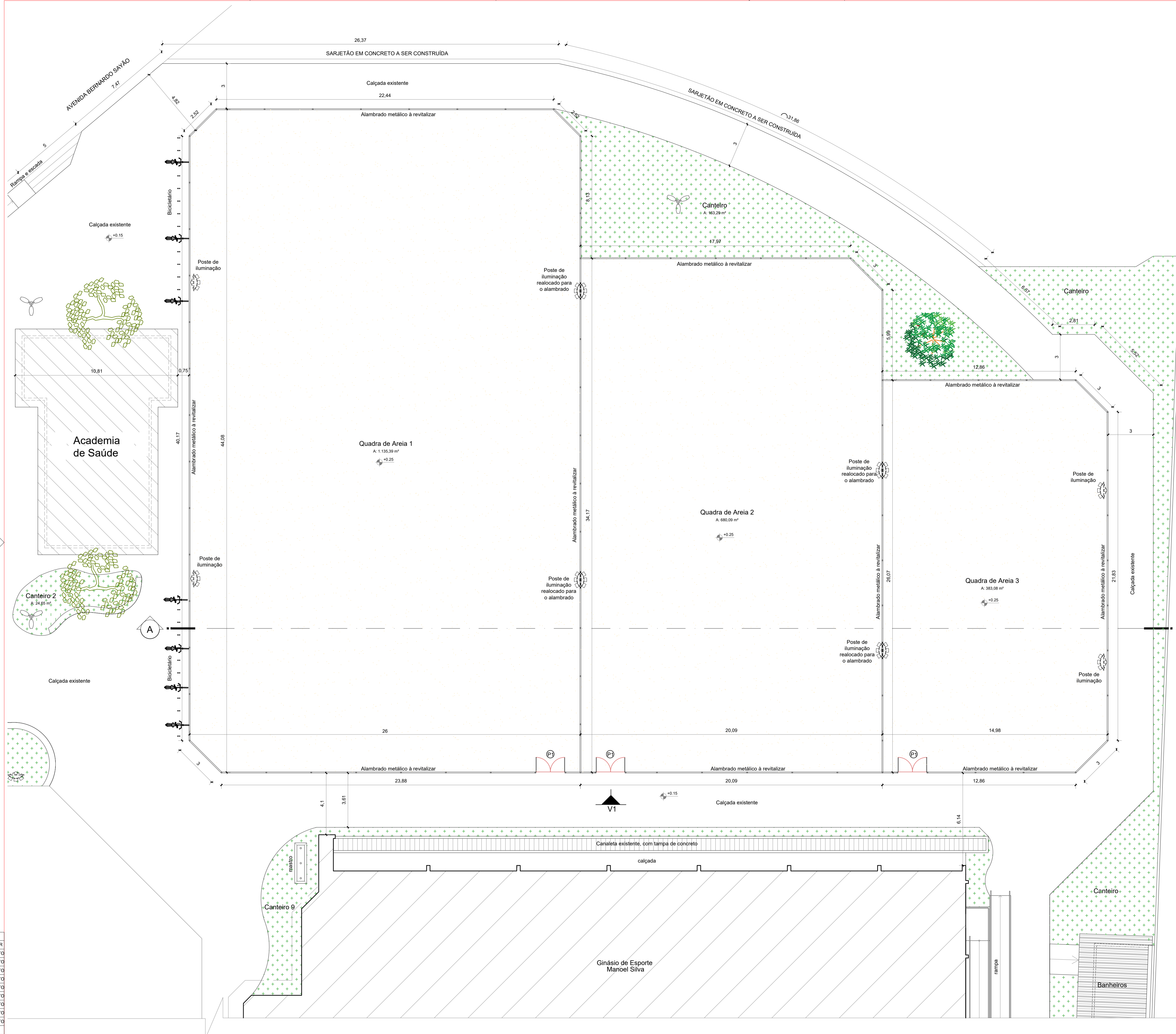
Planta Baixa Escala 1/125
