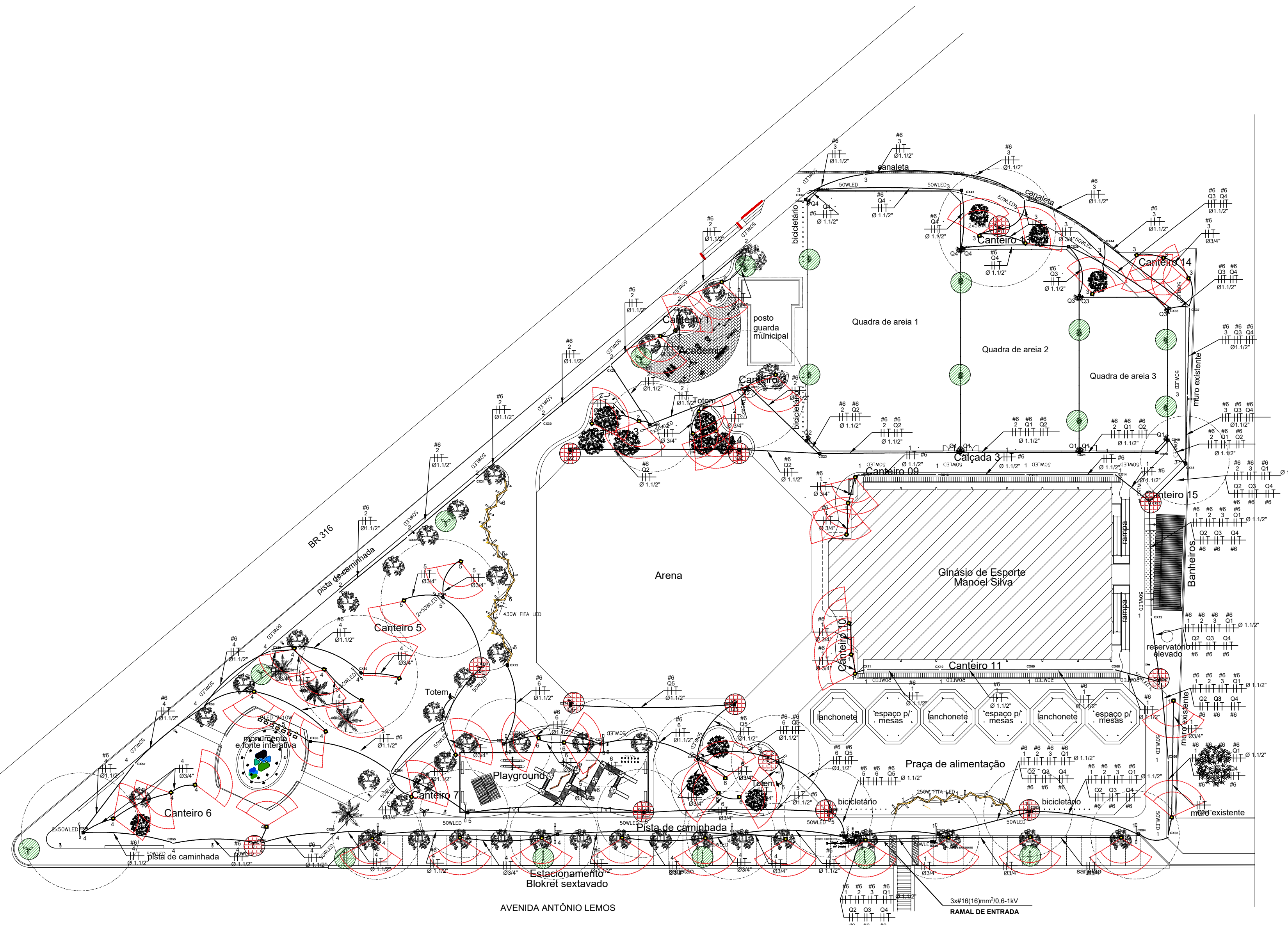
Planta Baixa Geral Escala 1/500
