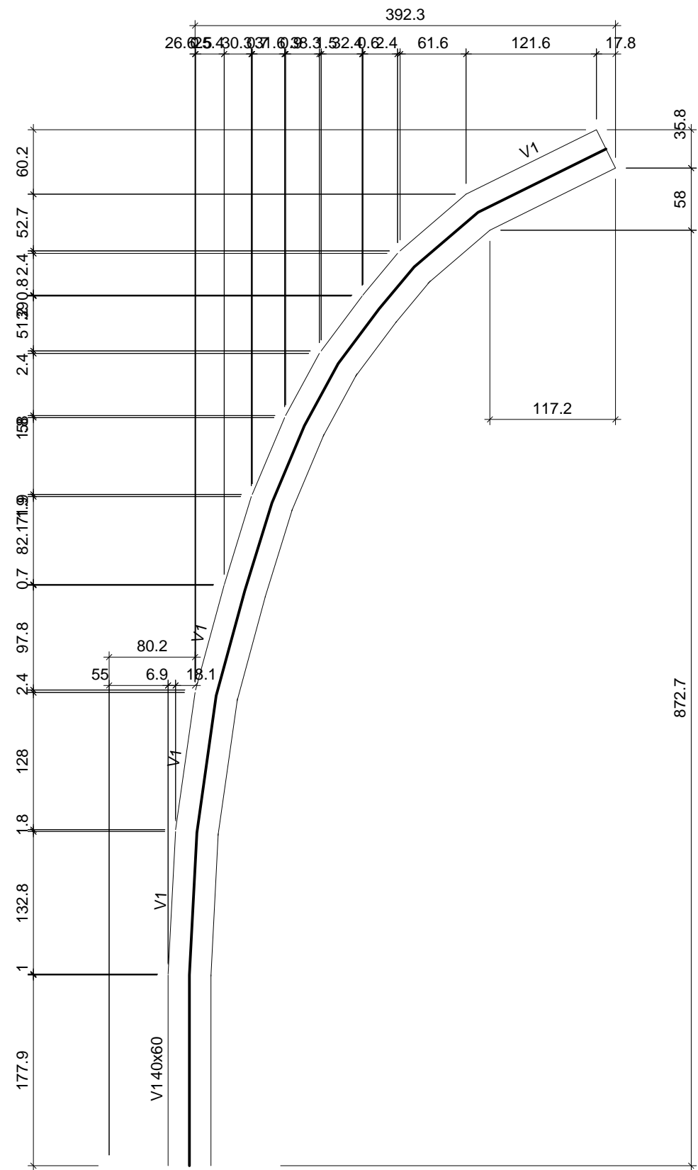
Forma Do Arco 01 Escala 1:50
