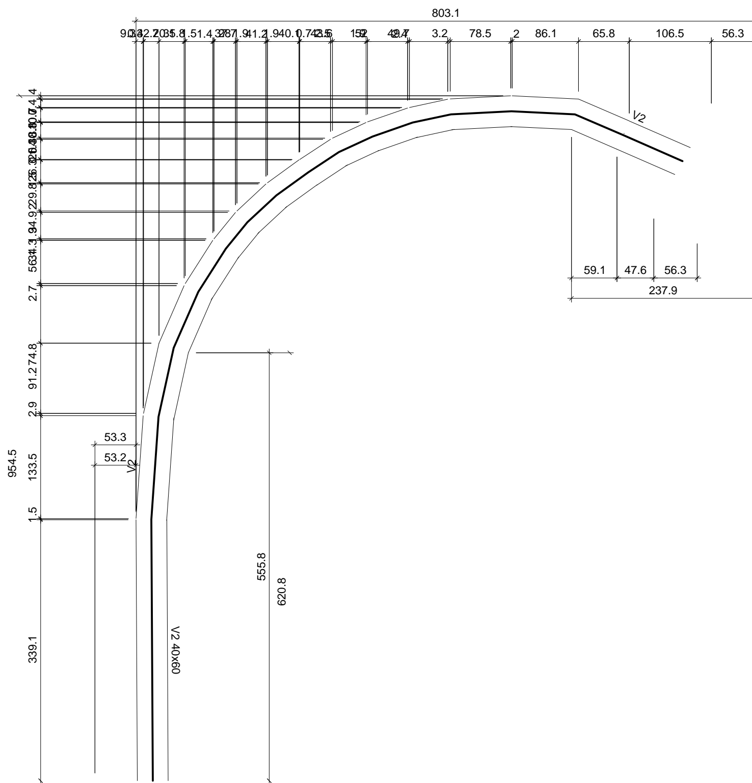
Forma Do Arco 02x2 Escala 1:50
