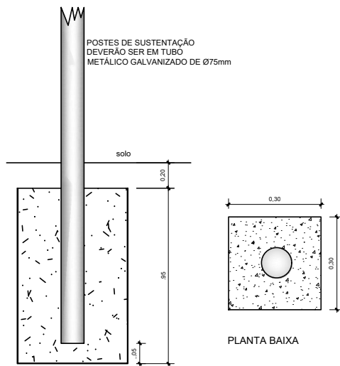
Detalhes do Bloco de Fundação
