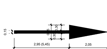
DETALHE DA SETA DE POSICIONAMENTO NA FAIXA
