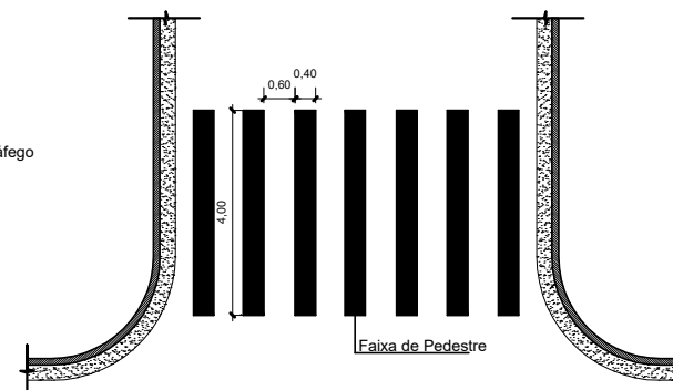
FAIXA DE PEDESTRE ZEBRADA
